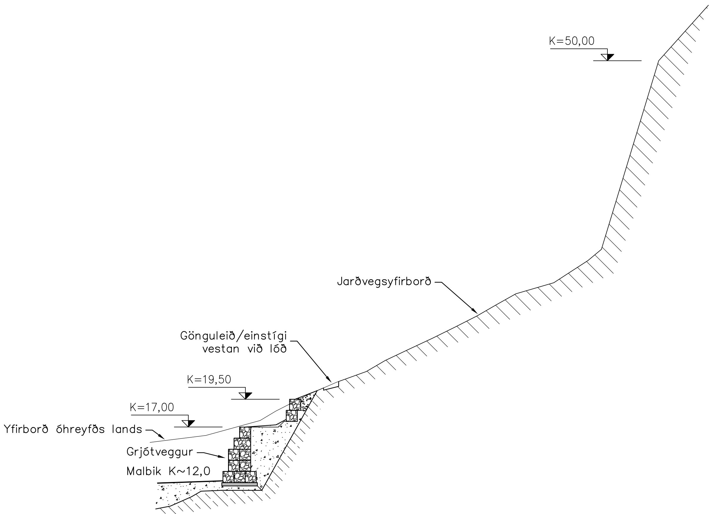
A 001 Þversnið – Grjótveggur og fjallshlíð vestan við lóð (Flatir) 1:200
